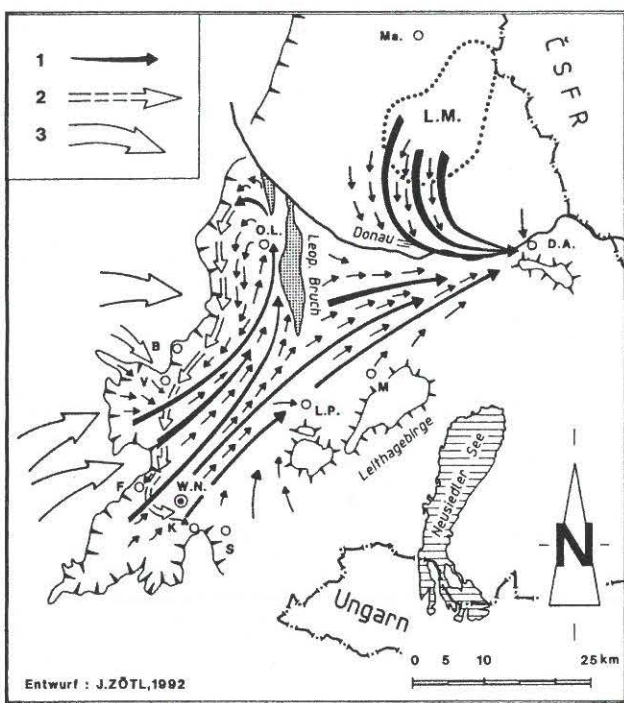
Schema der Tiefengrundwasser-Fließrichtungen
